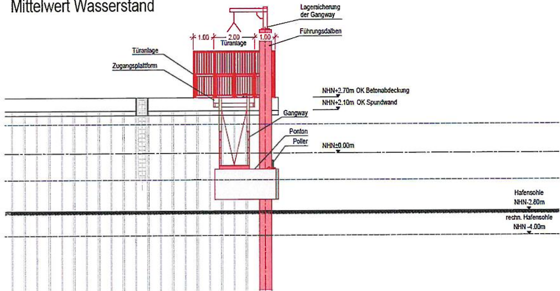
Abb. 11 Ansicht von der Wasserseite
