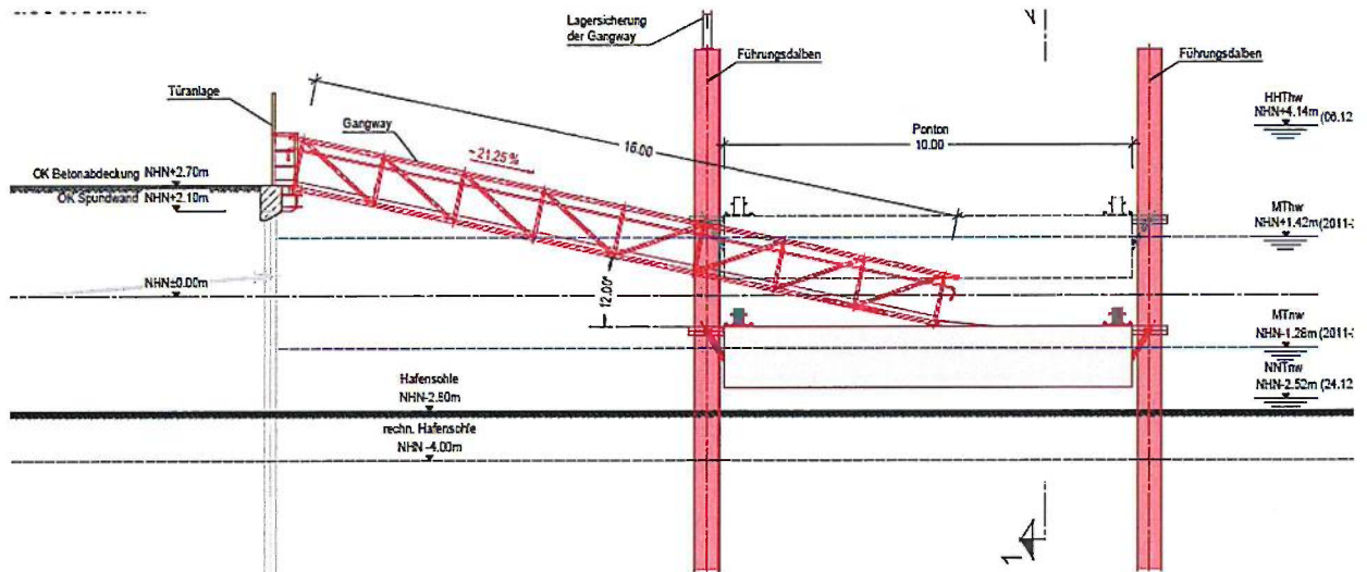
Abb. 8 Schnitt Anleger bei mittlerem Tideniedrigwasser
