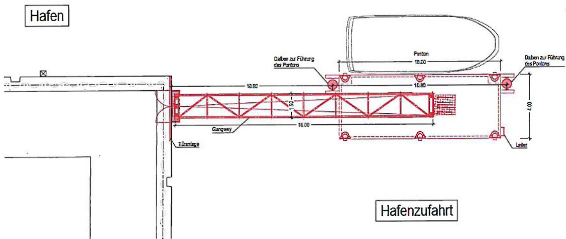
Abb. 12 Draufsicht neuer Anleger
