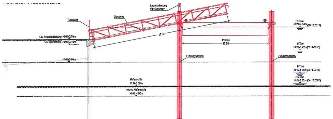
Abb. 9 Schnitt Anleger bei extremem Hochwasser
