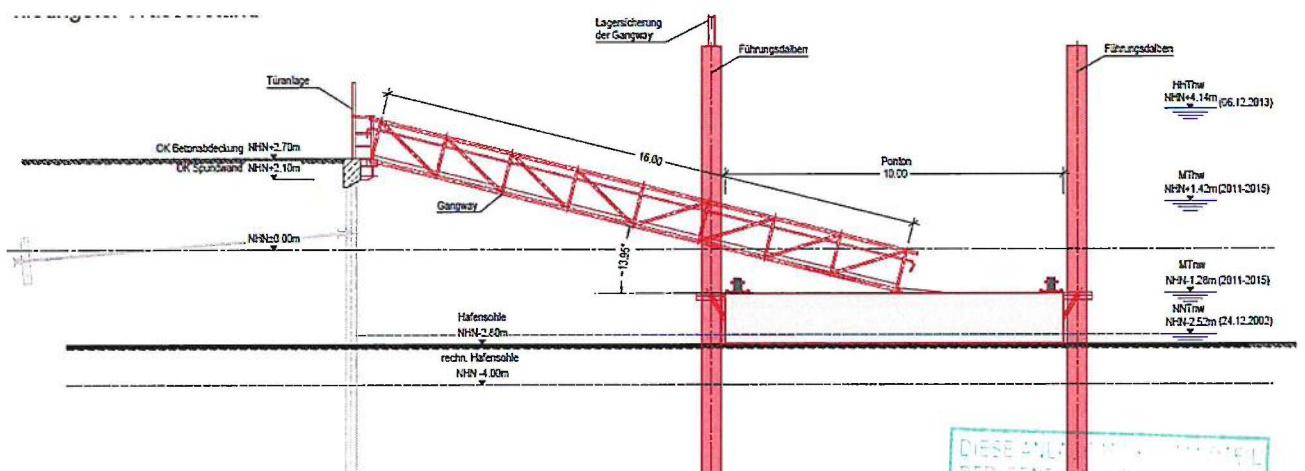
Abb. 10 Anleger bei extremem Niedrigwasser
